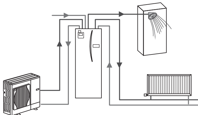
Pakettivaraajajärjestelmän kaavioesitys
